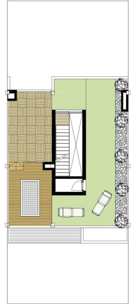
Planta Cubierta
