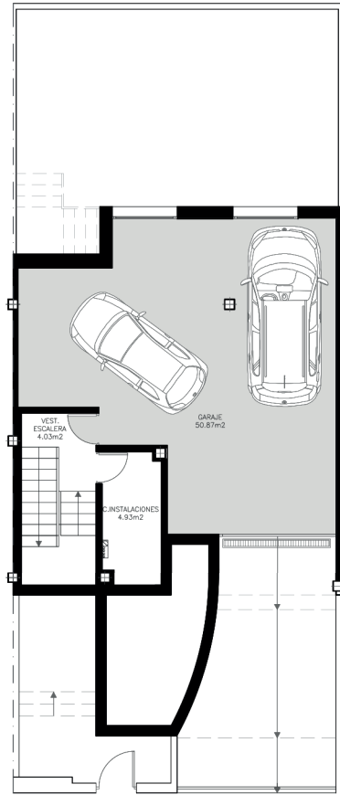
PLANTA SÓTANO
